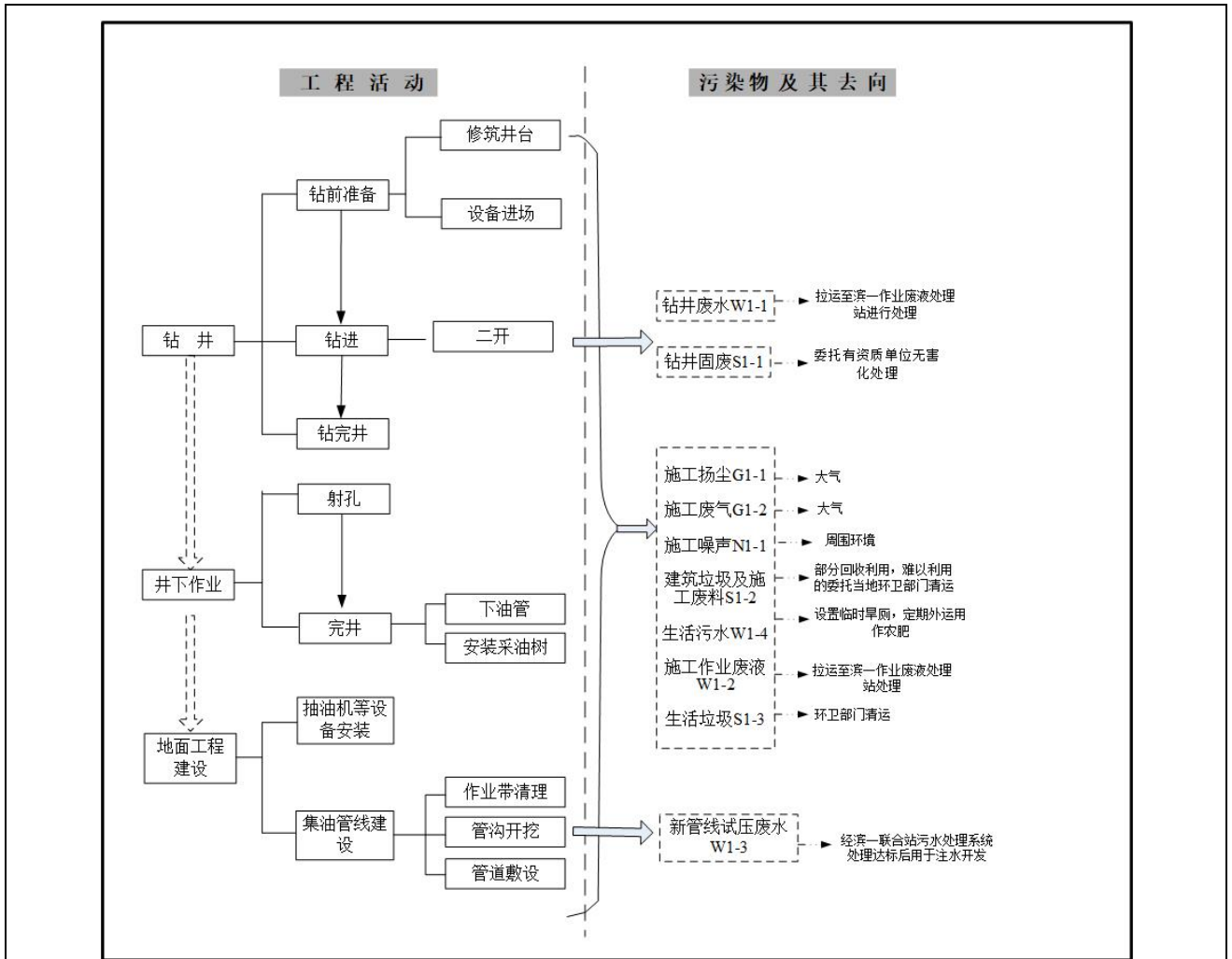
图 3-3 施工期工艺流程及产污环节图
