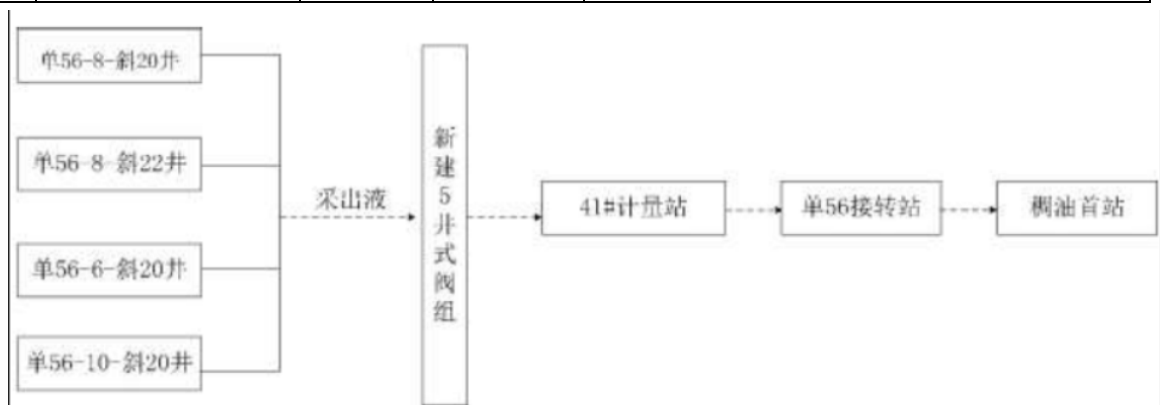
图 3-2 集输流程
